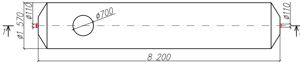
Вид сверху
