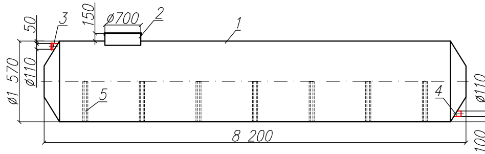
Разрез 1-1
