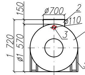
Вид спереди
